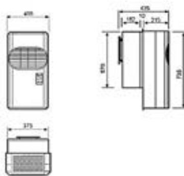
Wymiary dla serii RCV1
